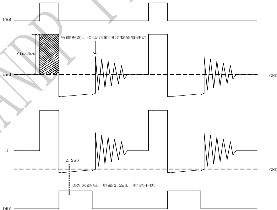
图 4 系统关键节点相对于 LP3510 的 GND 波形
