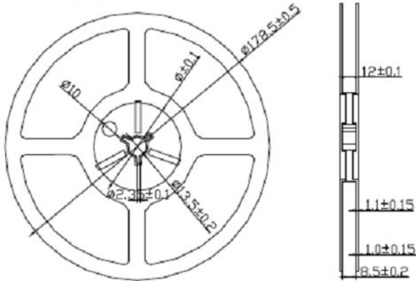
卷轴尺寸 Reel Dimension
