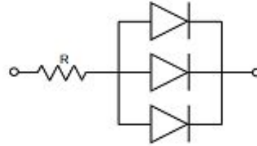
电路模式 B
