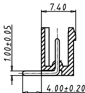
剖视图 A-A
