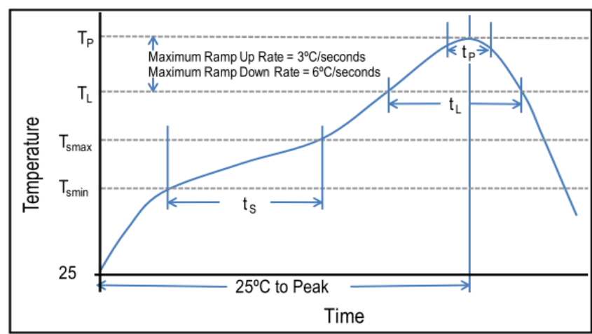
回流焊温度曲线
