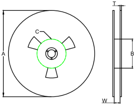
轮盘尺寸图
